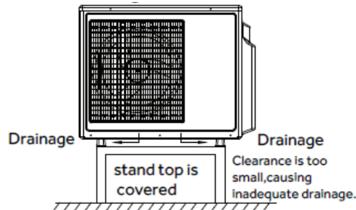
instalación incorrecta
