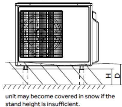
mauvaise installation
