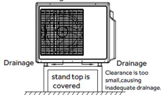
mauvaise installation
