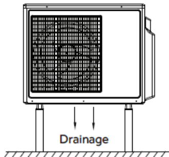
instalación correcta
