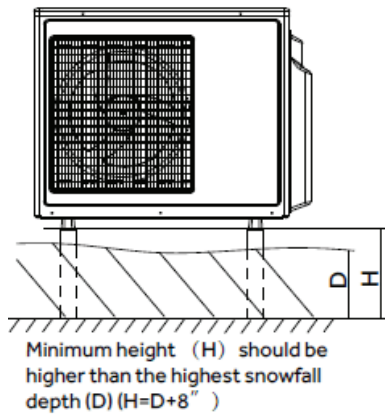
installation correcte
